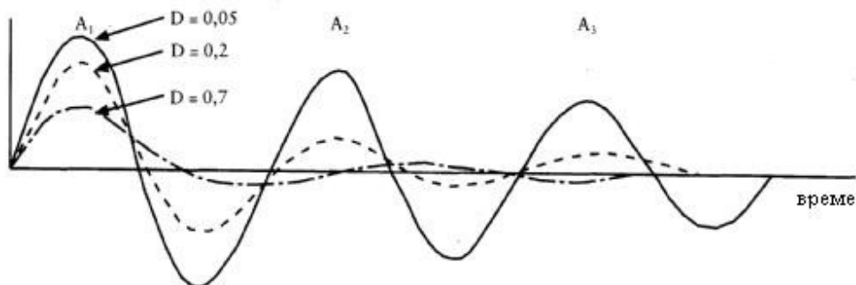
Фиг. 1. Синусоидална крива при свободни и краткотрайни трептения. Честотата може да бъде изчислена чрез измерване на времето до момента, в който цикличността на трептенето би могла да се забележи. Затихването може да бъде изчислено, като се
