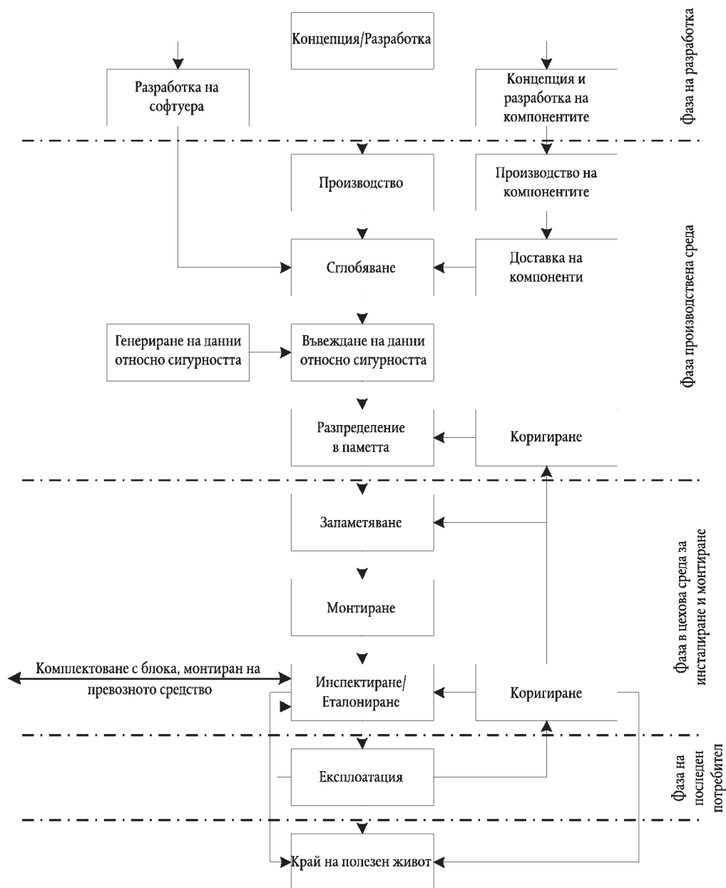
Характерен цикъл на живот на датчика за движение
