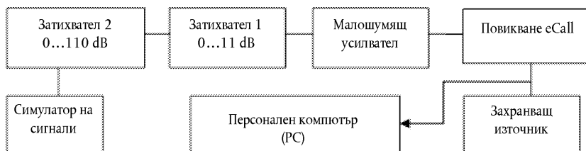
Схема за оценка на чувствителността на модул за ГНСС
