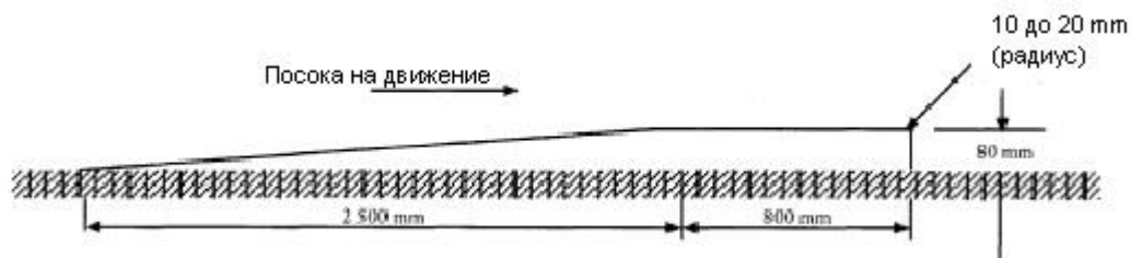
Фиг. 2. Праг за изпитване на окачването За извършване на измерв
